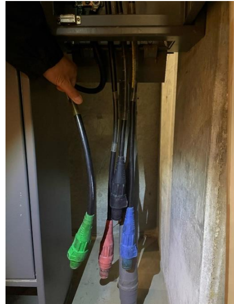
大ホール照明用仮設電源 200V 3相3線
